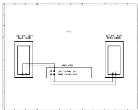
Installation des enceintes EZY SAT sans caisson actif EZY SUB Installation of EZY SAT without EZY SUB subwoofer (figure 1)
